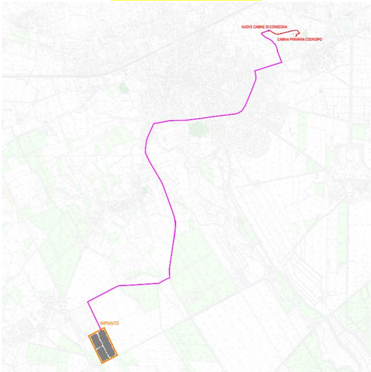
Immagine 5.3.3: Percorso cavidotto MT su CTR (Alternativa 2)
